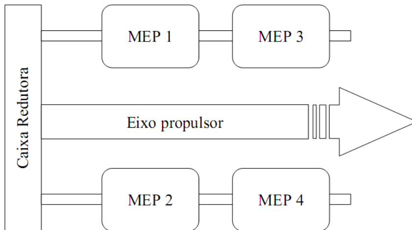
Figura 14: Esquema de propulsão em corrente contínua com quatro MEPs.
