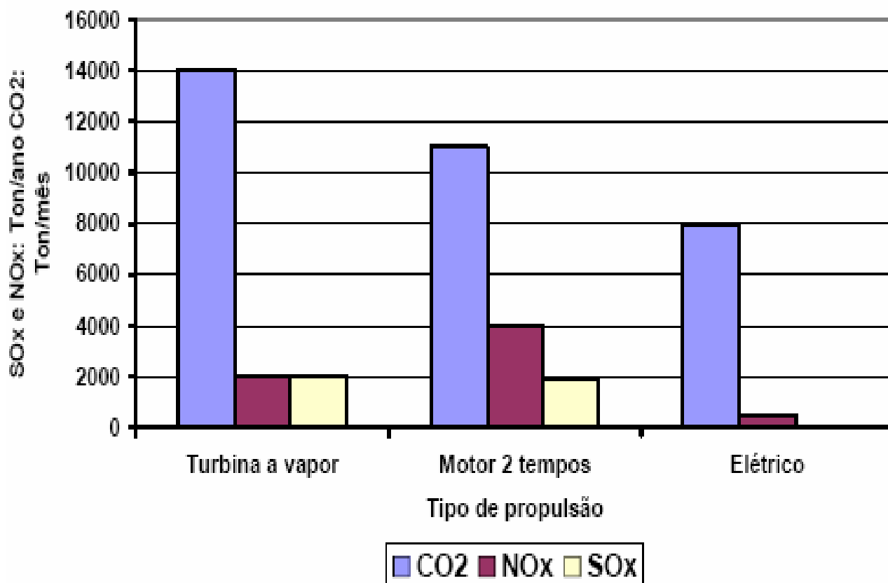
Figura 18: Gráfico comparativo das emissões de gases para a atmosfera.
