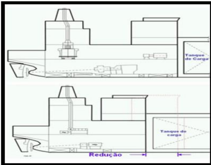
Figura 17: Distribuição dos equipamentos na Praça de Máquinas.
