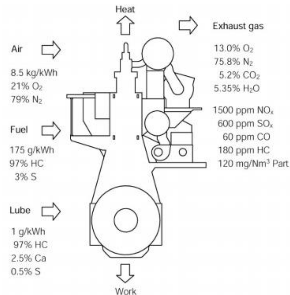
Figura 5: Valores típicos dos poluentes emitidos para a atmosfera por um motor diesel marítimo.
