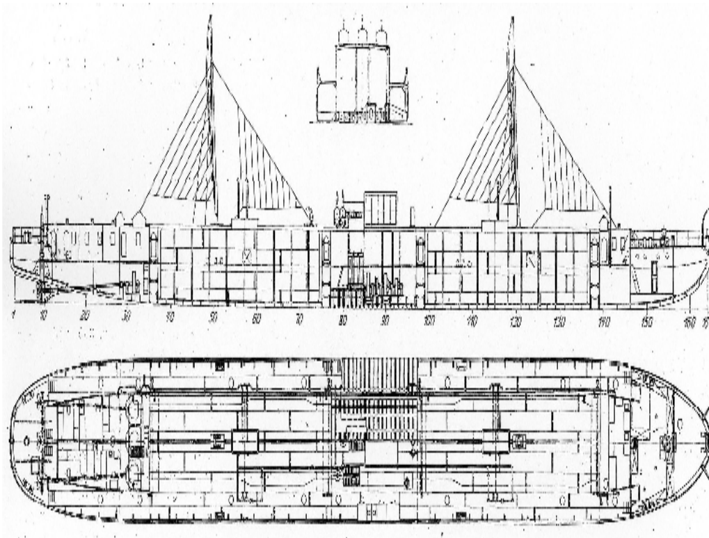
Figura 8: Plano de perfil e superior do Vandal (tanker).
