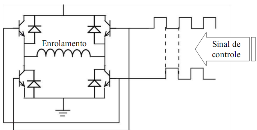
Figura 15: Esquema básico do ligação de um dos enrolamentos de um motor propulsor em corrente alternada com inversor.
