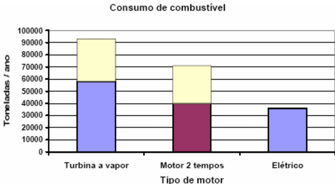
Figura 16: Gráfico comparativo de consumo de combustível.
